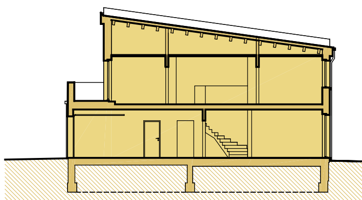
řez domu A-A
